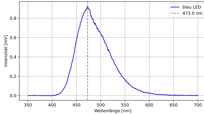
Abbildung 12: Spektrum der blau leuchtenden Diode mit einem Maximum bei 473,0 nm.
