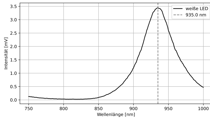
Abbildung 17: Optional gemessenes Infrarotspektrum der weißen LED mit einem Maximum bei 935,0 nm.
