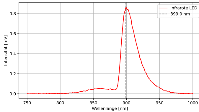
Abbildung 16: Spektrum der Infrarot emittierenden GaAs-Diode mit einem Maximum bei 899,0 nm.
